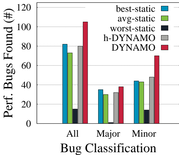
Figure 8: m-PetStore
