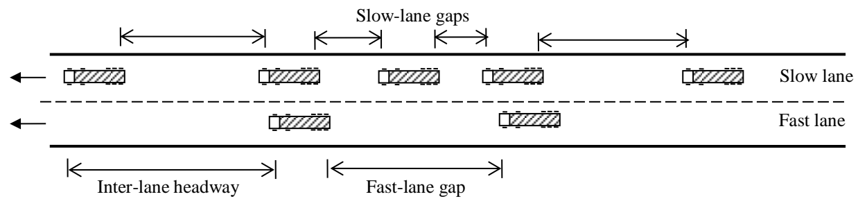
Fig. 1. Traffic scenario.
