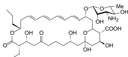
6 Rimocidin
