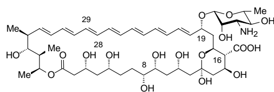
2 Amphotericin B
