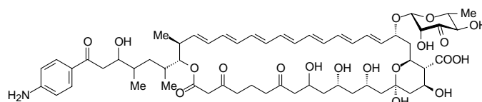
32 FR008-XI
