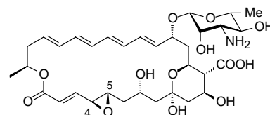
4 Pimaricin
