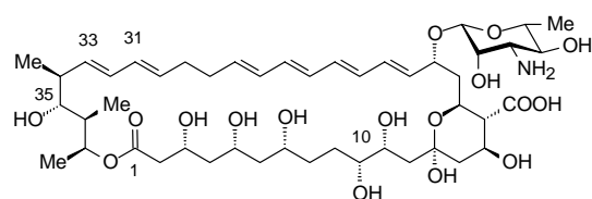
1 Nystatin A1
